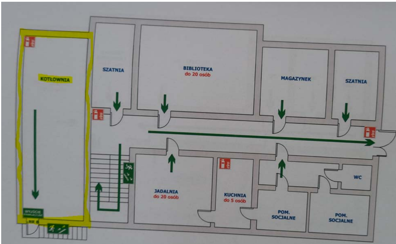
Rys. lokalizacja pomieszczenia kotłowni na poziomie -1
