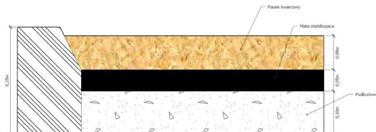
Układ warstw podłoża jeździeckiego
