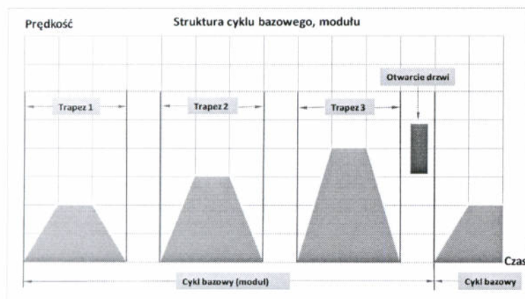
Rys. 1. Struktura cyklu bazowego SORT.
