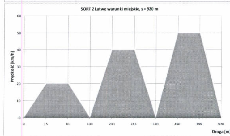
Rys. 3. Struktura cyklu SORT 2.
