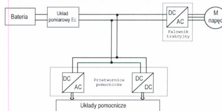
Rys. 5. Miejsca pomiaru energii elektrycznej.
