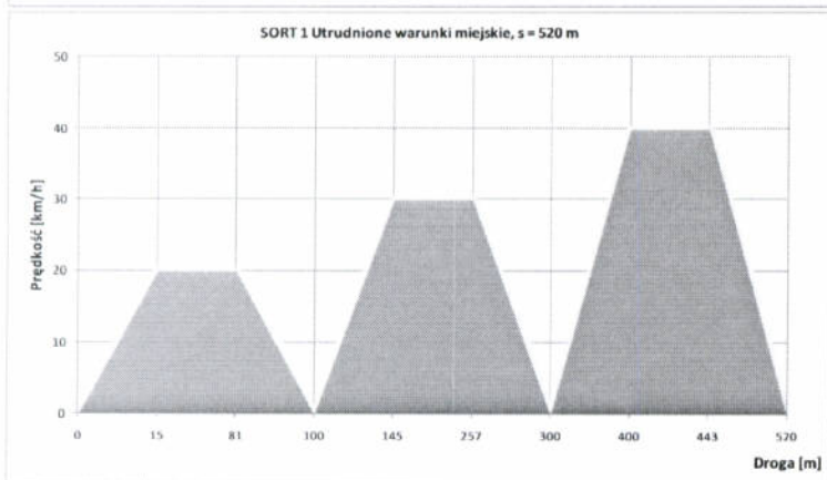
Rys. 2. Struktura cyklu SORT 1.
