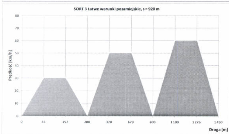
Rys. 4. Struktura cyklu SORT 3.
