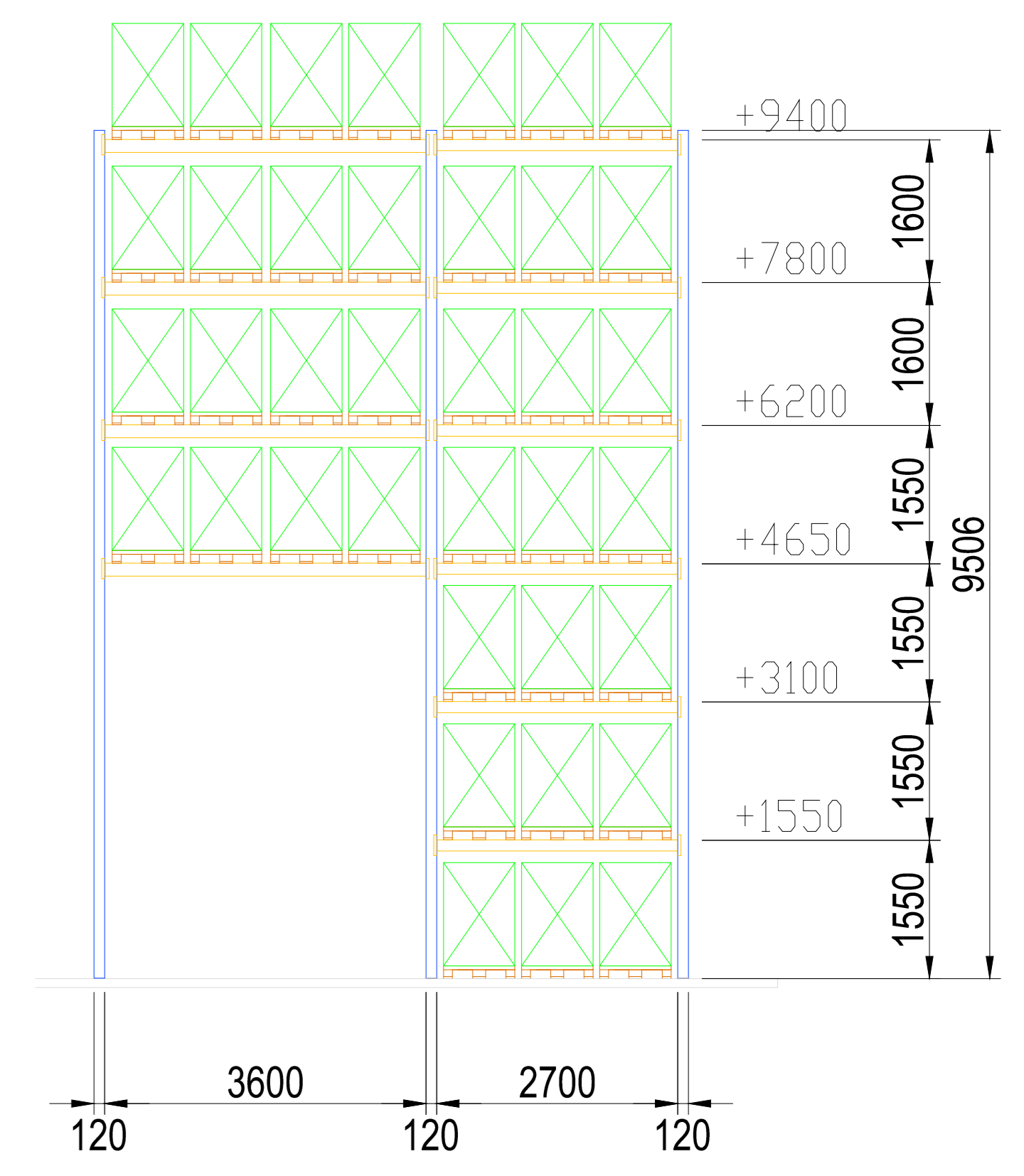
Układ poziomów składowania
