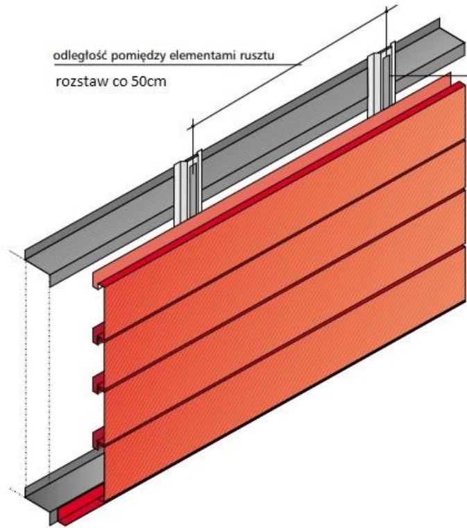
Profil Omega gr. blachy 2,5mm
