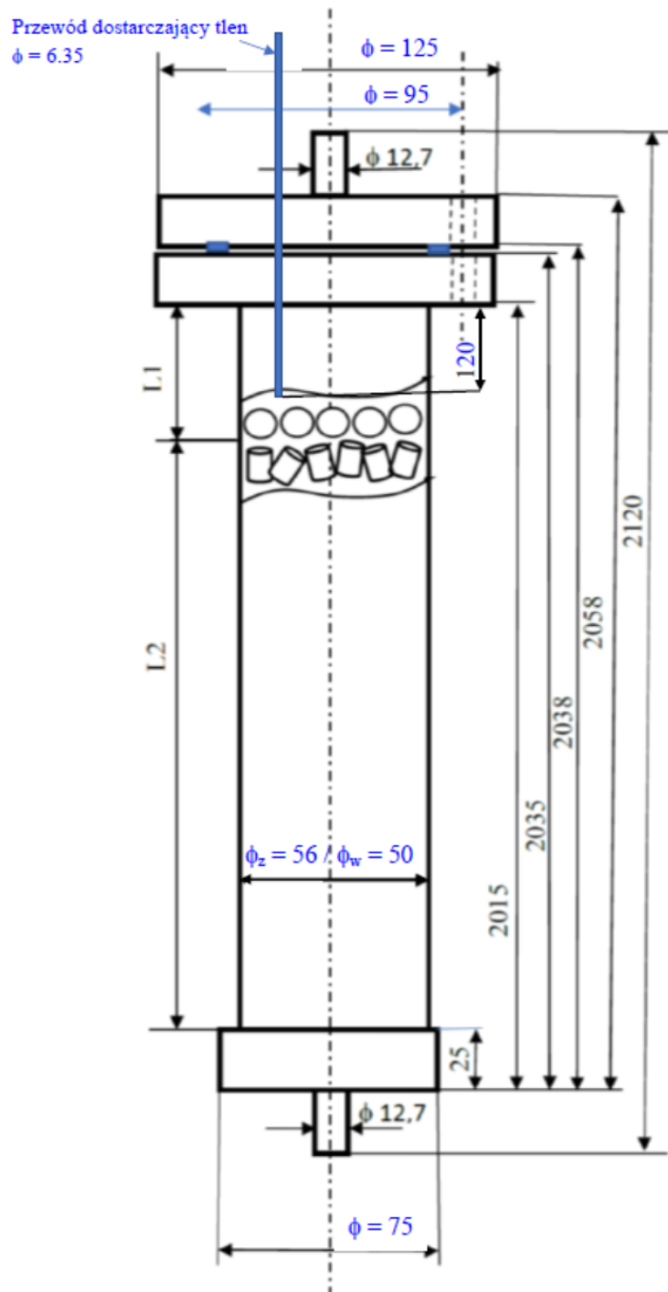
Rys. 2. Schemat pojedynczego reaktora zamontowanego w korpusie reformera
