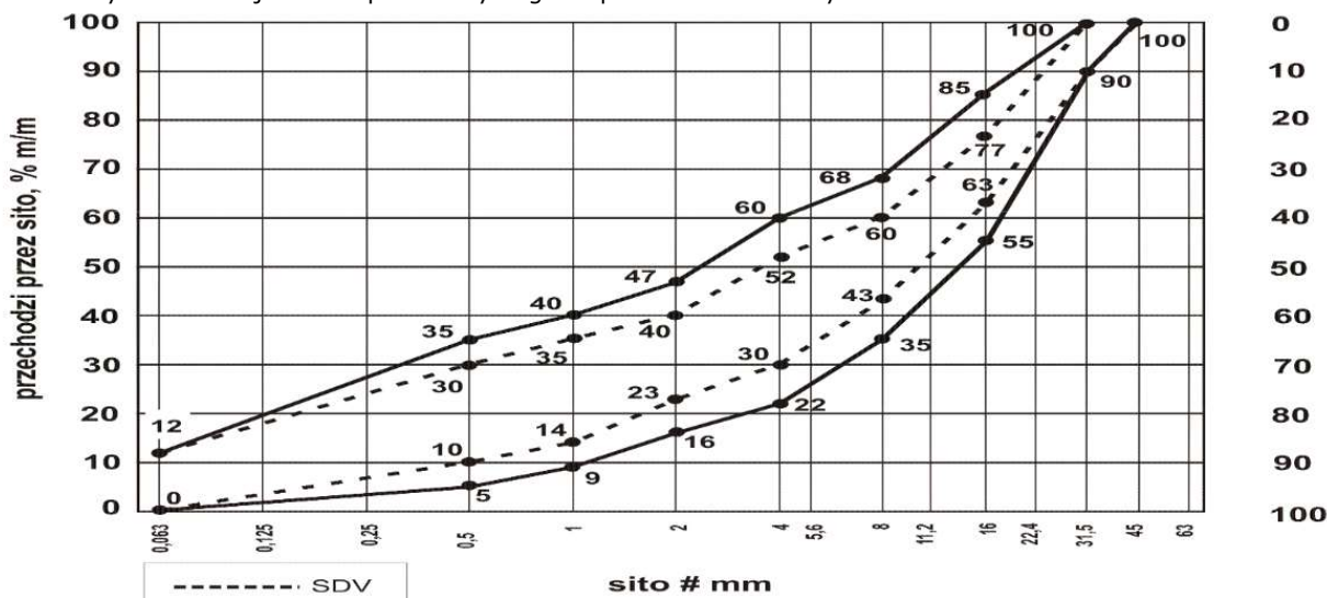
Rysunek 1. Mieszanka niezwiązana 0/31,5
