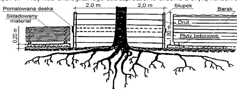
Rys. 6. Przykład ekologicznego zabezpieczenia drzewa z bryłą korzeniową na placu składowym (wg [10])
