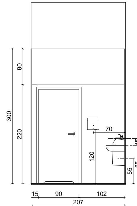
ŚCIANA D_E
