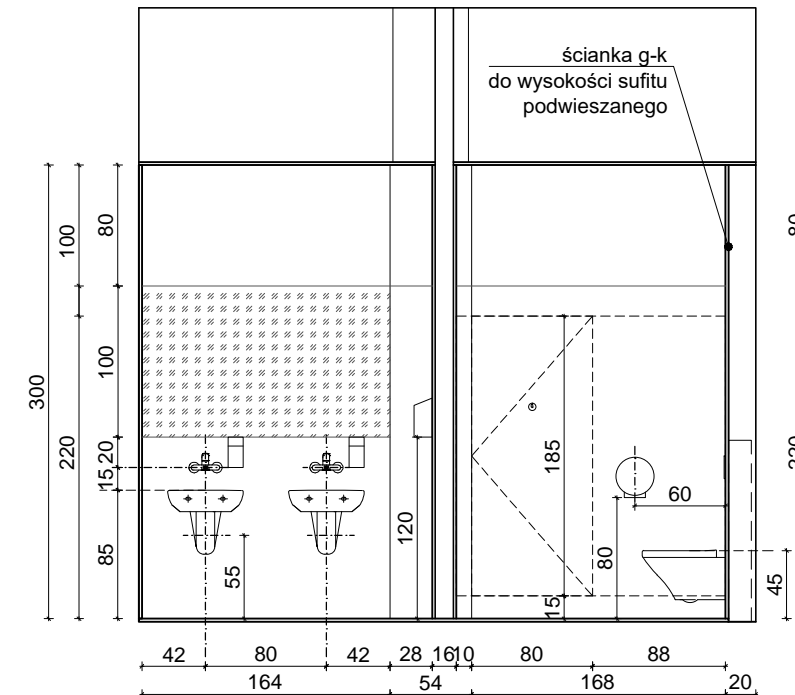
ŚCIANA E_A
