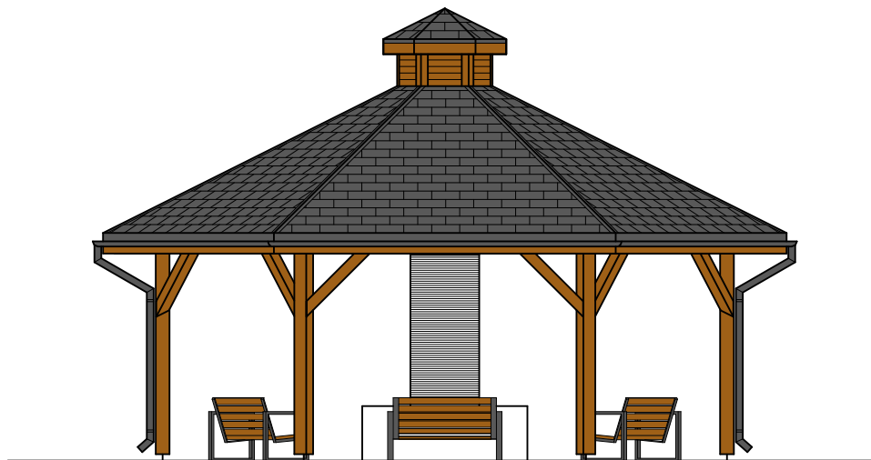
Elewacja północna
