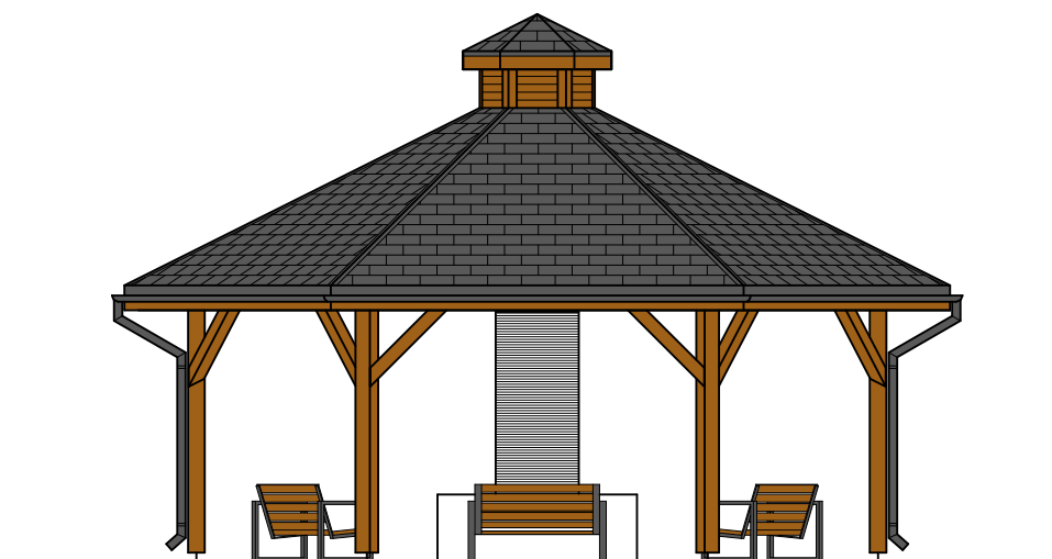
Elewacja południowa
