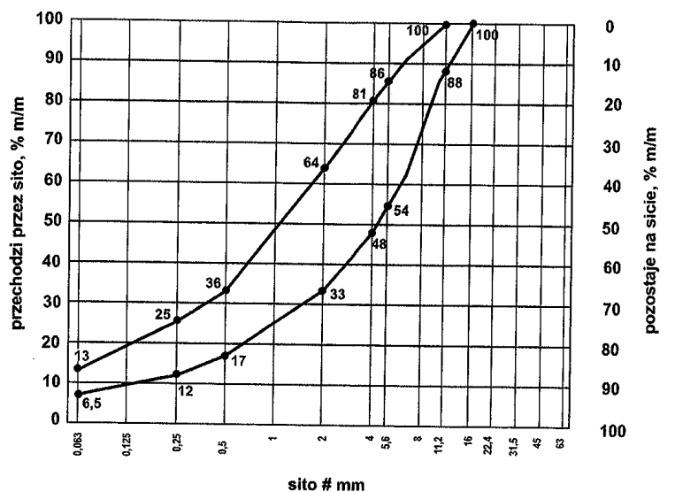
Rys. 3. Krzywe graniczne uziarnienia mieszanki zawiązanej spoiwem drogowym typu 2 o uziarnieniu 0/16 mm
