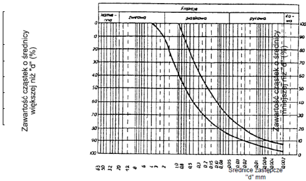
Rysunek 1. Obszar uziarnienia optymalnej mieszanki gliniasto-piaskowej
