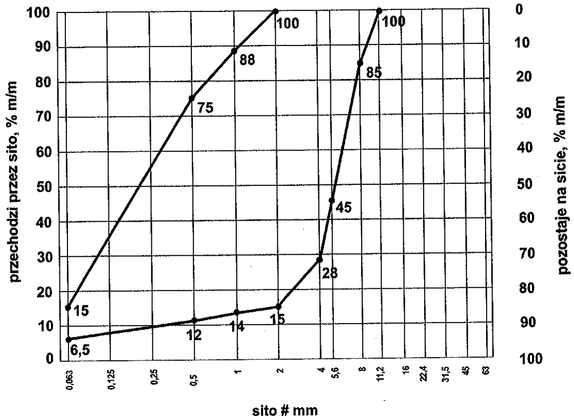
Rys. 2 uziarnienie mieszanki 0/11,2
