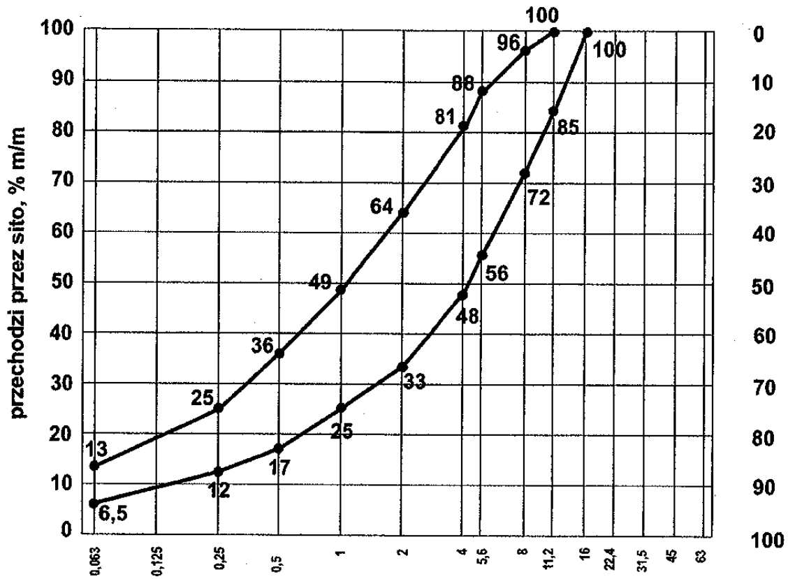
Rys. 3 uziarnienie mieszanki 0/16
