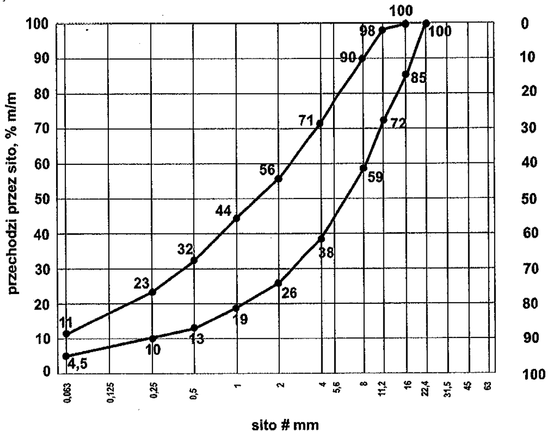
Rys. 3 uziarnienie mieszanki 0/16
