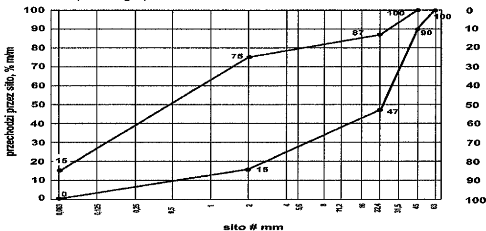
Rys. 6. Krzywe graniczne uziarnienia mieszanki kruszyw 0/45 mm do górnej warstwy ulepszonego podłoża
