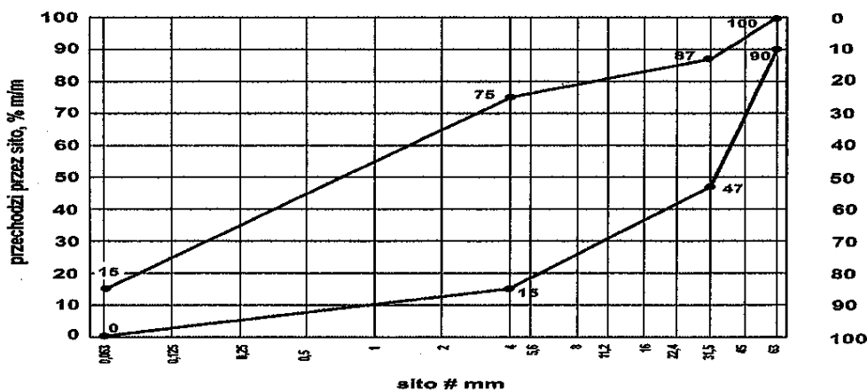
Rys. 7. Krzywe graniczne uziarnienia mieszanki kruszyw 0/63 mm do górnej warstwy ulepszonego podłoża
