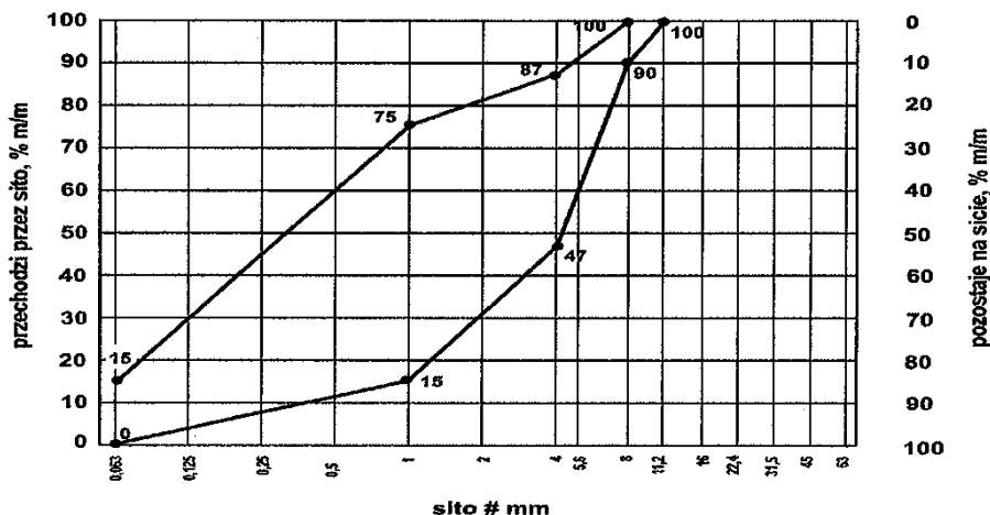
Rys. 1. Krzywe graniczne uziarnienia mieszanki kruszyw 0/8 mm do górnej warstwy ulepszanego podłoża
