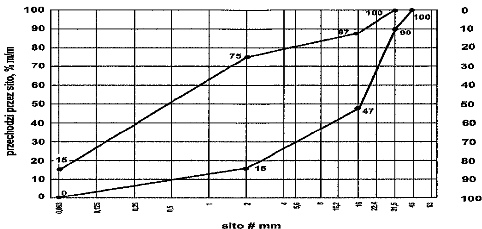
Rys. 5. Krzywe graniczne uziarnienia mieszanki kruszyw 0/31,5 mm do górnej warstwy ulepszonego podłoża
