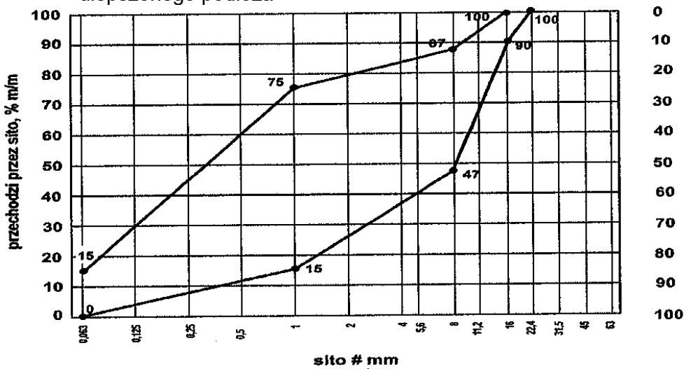
Rys. 3. Krzywe graniczne uziarnienia mieszanki kruszyw 0/16 mm do górnej warstwy ulepszonego podłoża
