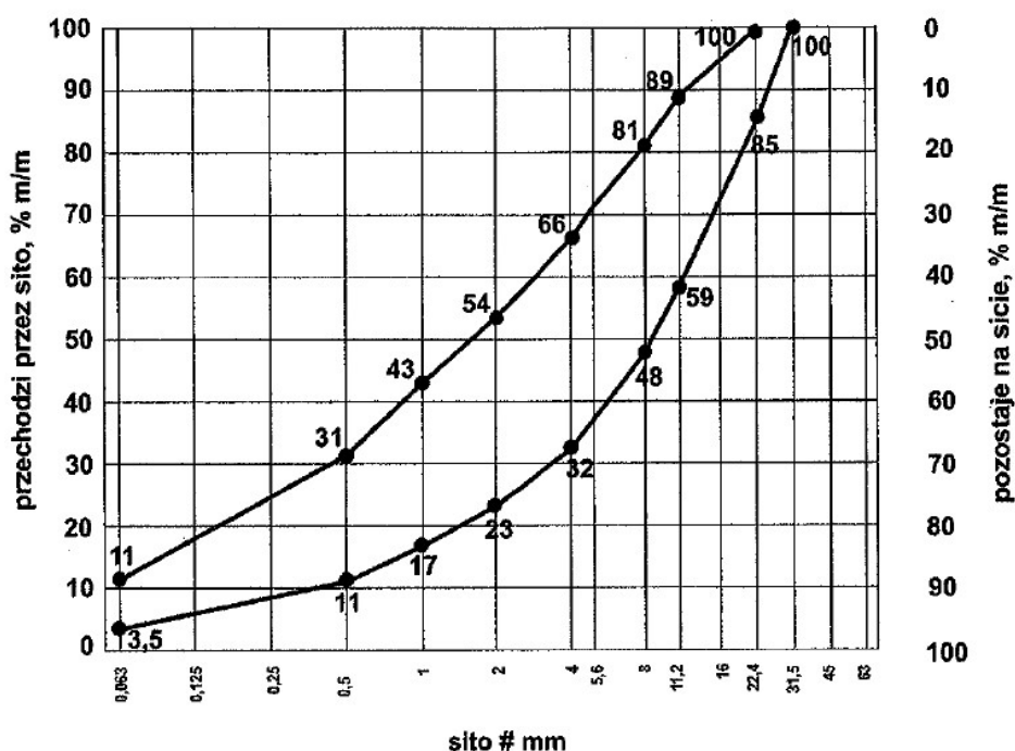
Mieszanka 0/22,4
