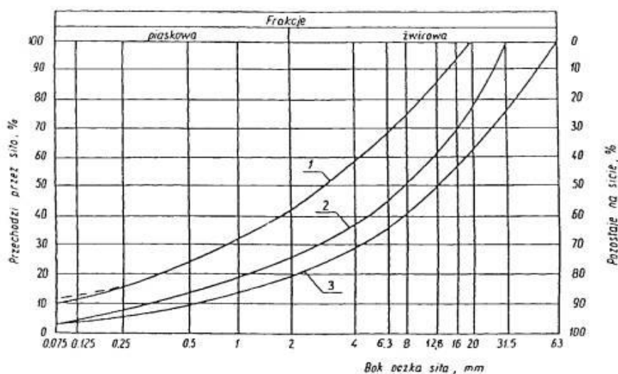
Rys. 2. Uziarnienie mieszanki niezwiązanej 0/31,5 dla podbudowy pomocniczej
