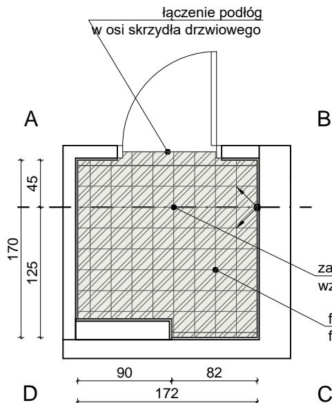
RZUT POSADZKI
