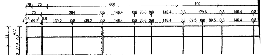
ELEWACJA - KURKOWA
