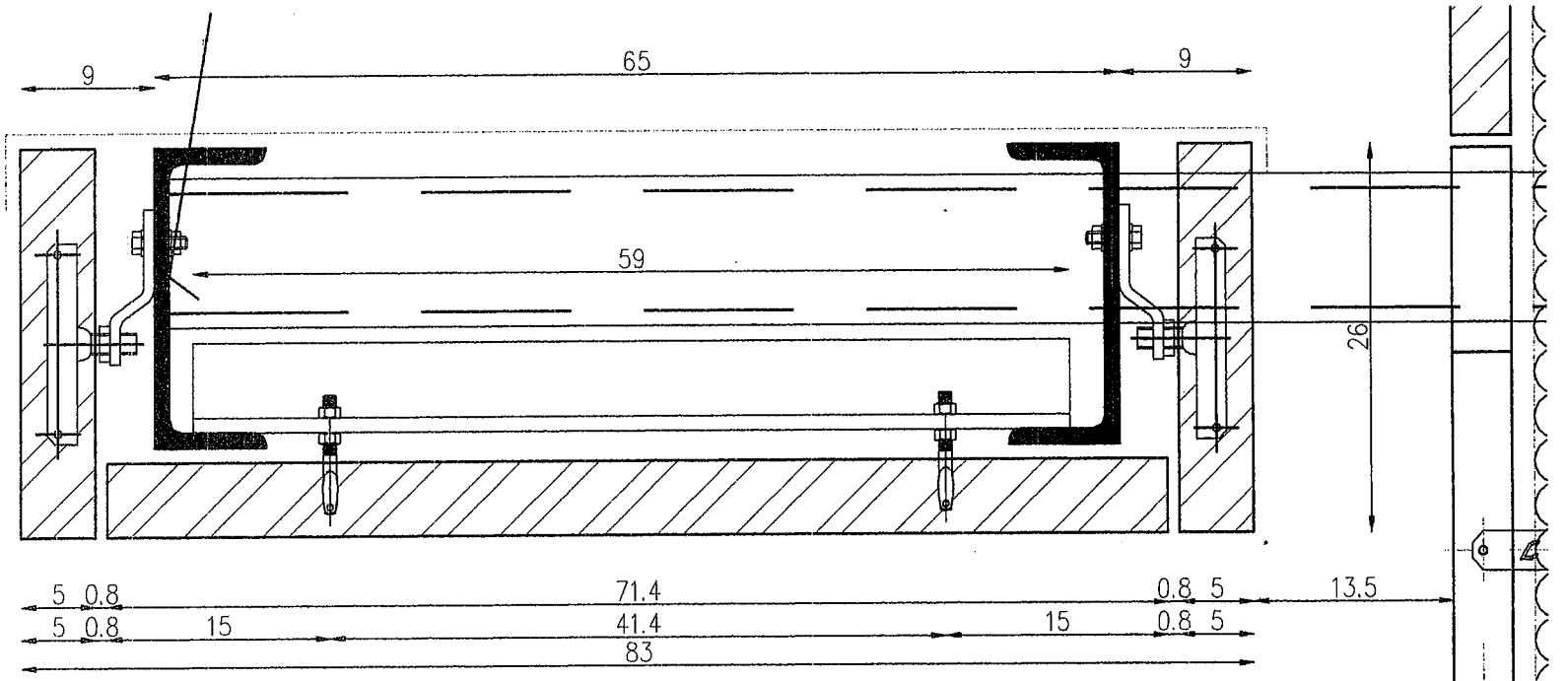
ELEWACJA - KURKOWA
