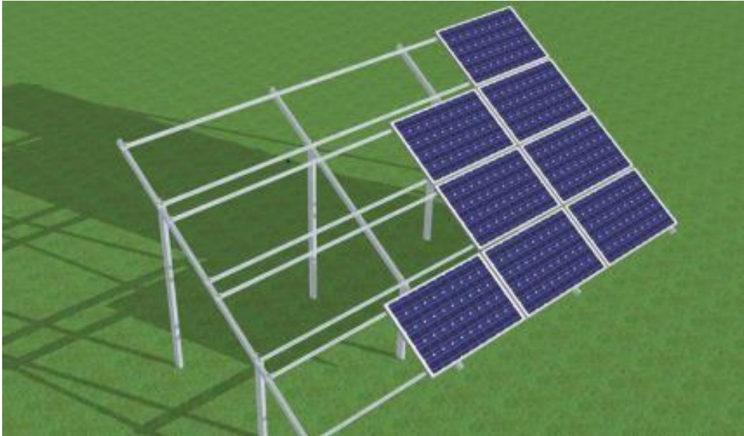
Rysunek 28 - Poglądowy szkic konstrukcji naziemnej
