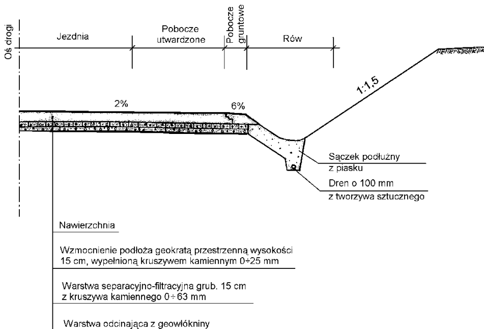
Rys. 4. Przekrój poprzeczny drogi ze wzmocnieniem podłoża geokratą i kruszywem kamiennym
