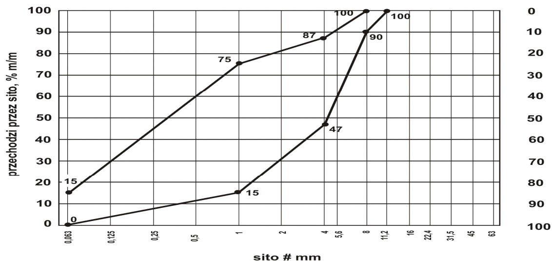
Rys. 1. Uziarnienie mieszanki niezwiązanej 0/8 dla nawierzchni
