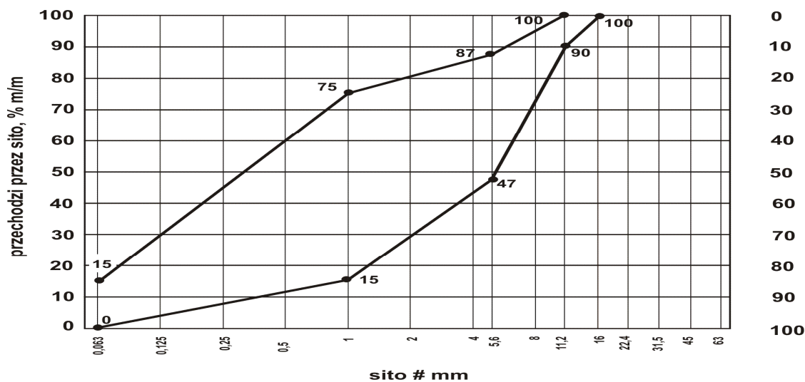
Rys. 2. Uziarnienie mieszanki niezwiązanej na 0/11,2 dla nawierzchni
