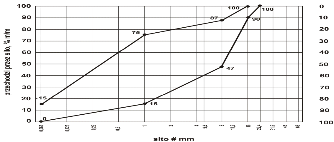
Rys. 3. Uziarnienie mieszanki niezwiązanej 0/16 dla nawierzchni
