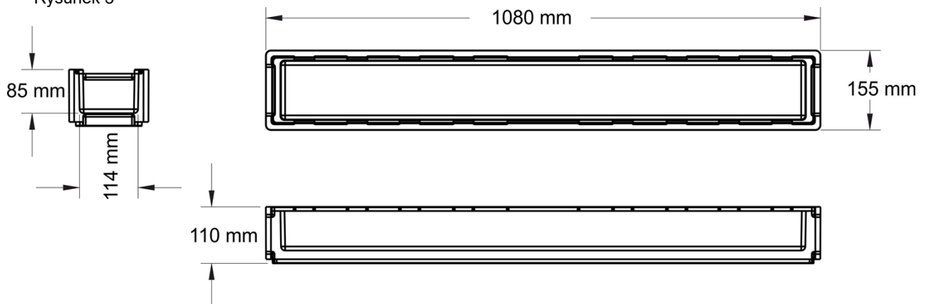
Szkic opakowania styropianowego do przechowywania 1/2 części rdzenia o średnicy max 114 mm
