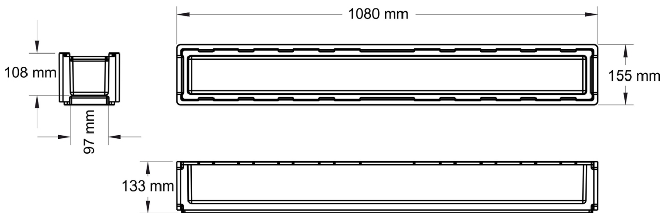
Szkic opakowania styropianowego do przechowywania pełnego rdzenia o średnicy max 97 mm
