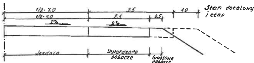
Rys. 3. Konstrukcja nawierzchni utwardzonego pobocza
