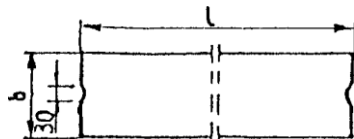
Rys. 1. Wymiarowanie krawężników
