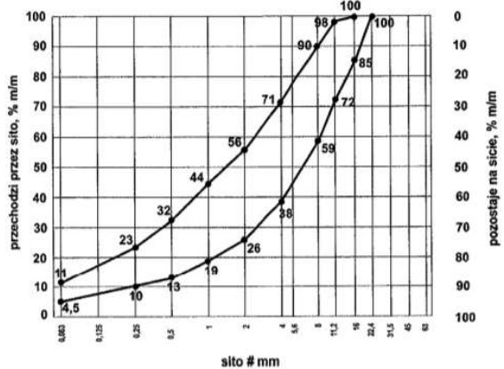
Rys. 3. Krzywe graniczne uziarnienia mieszanki mineralnej 0/16 mm
