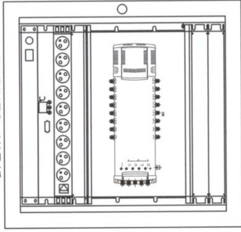
Szafka 19" 600x600 12U drzwi szklane
