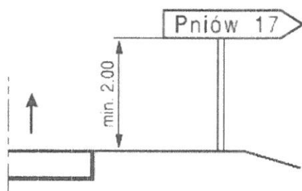
Rys. 6. Wysokość umieszczenia znaków E-3 na drogach
