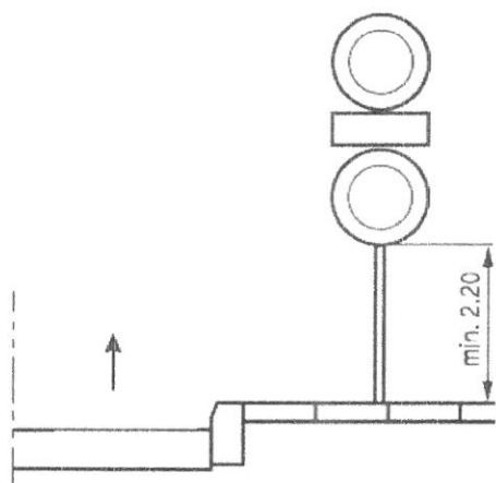
Rys. 5. Wysokość umieszczenia dwóch lub więcej znaków na jednym słupku na ulicach
