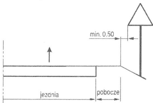
Rys. 1. Lokalizacja znaków od krawędzi jezdni na drodze
