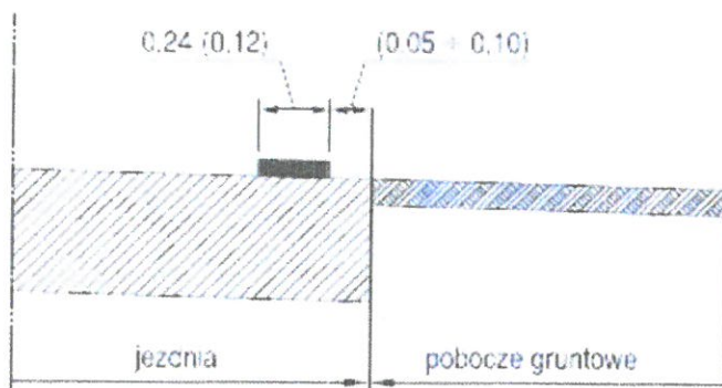
Rys. 8. Usytuowanie linii krawędziowej na jezdni z poboczem gruntowym
