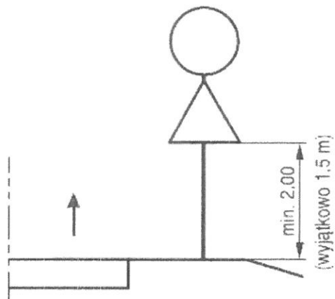
Rys. 7. Wysokość umieszczenia znaków dwóch znaków na jednym słupku na drogach innych niż ulice
