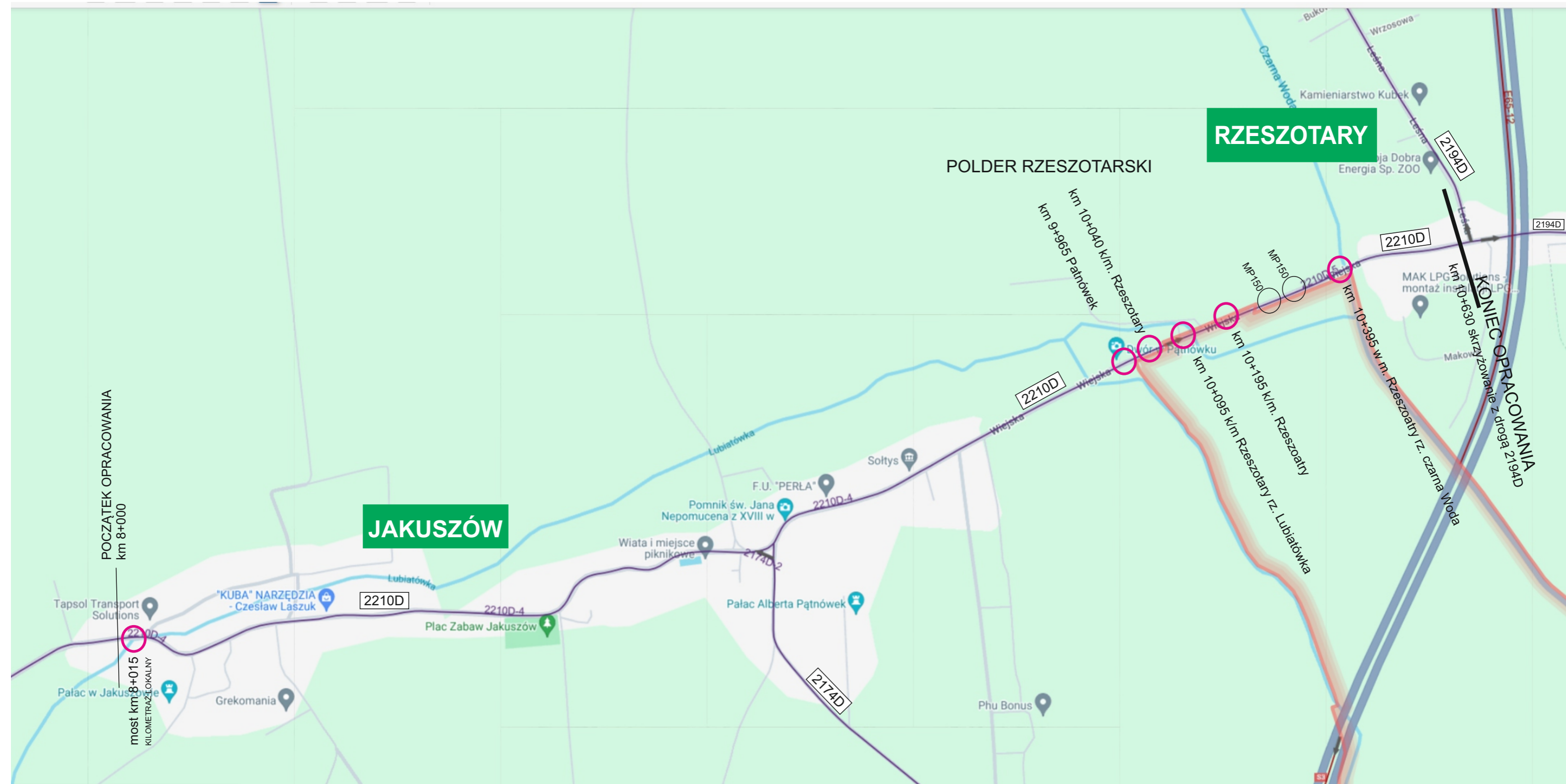
PLAN SYTUACYJNY dla zadania pn.: „Przebudowa i rozbudowa drogi powiatowej nr 2210D Jakuszów - Rzeszotary”
