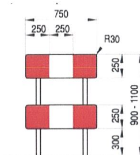
Ryc. 4 Typoszeręg wymiarów zapór drogowych U-20c:
