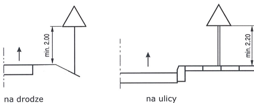
Ryc. 3 Wysokość umieszczenia znaków:
