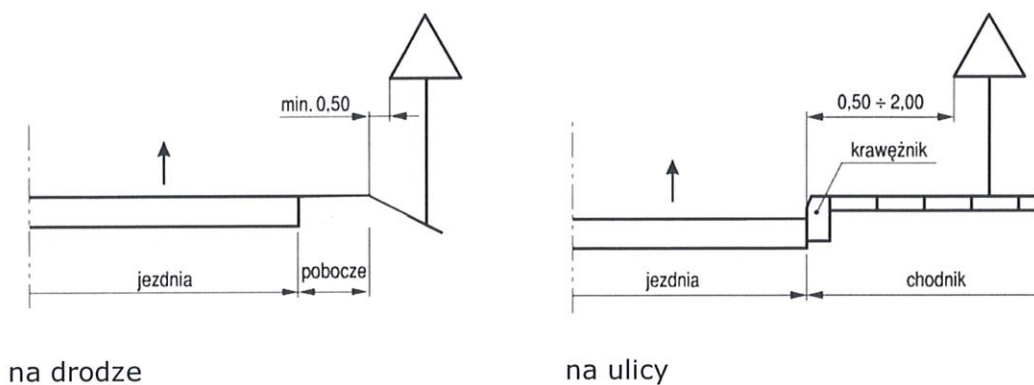
Ryc. 3 Wysokość umieszczenia znaków:
