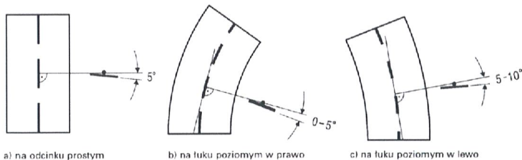
Ryc. 1 Odchylenie tarczy znaku
