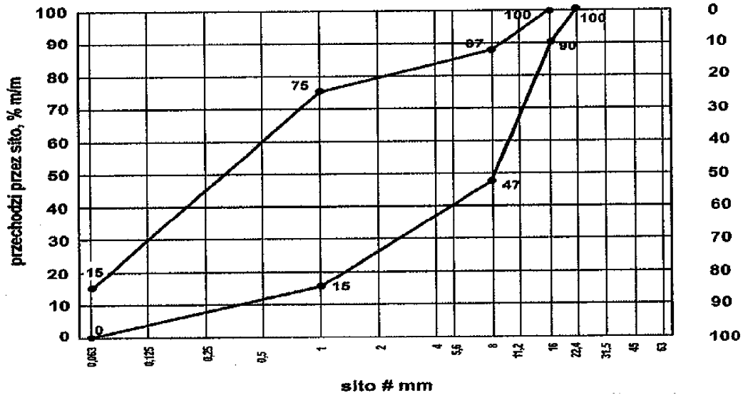
Uziarnienie mieszanki niezwiązanej 0/16 dla warstwy mrozoochronnej
