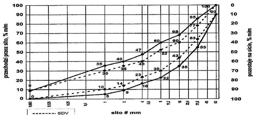
Rys. 14. Mieszanka niezwiązana 0/63 do warstw podbudowy zasadniczej
