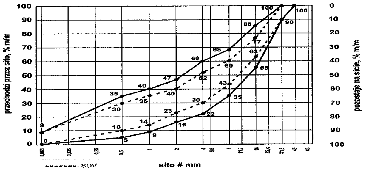
Rys 1 Mieszanka niezwiązana 0/31,5
