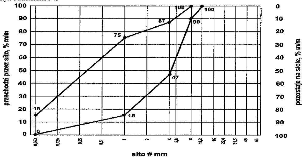
Rys. 9 Mieszanka 0/63
