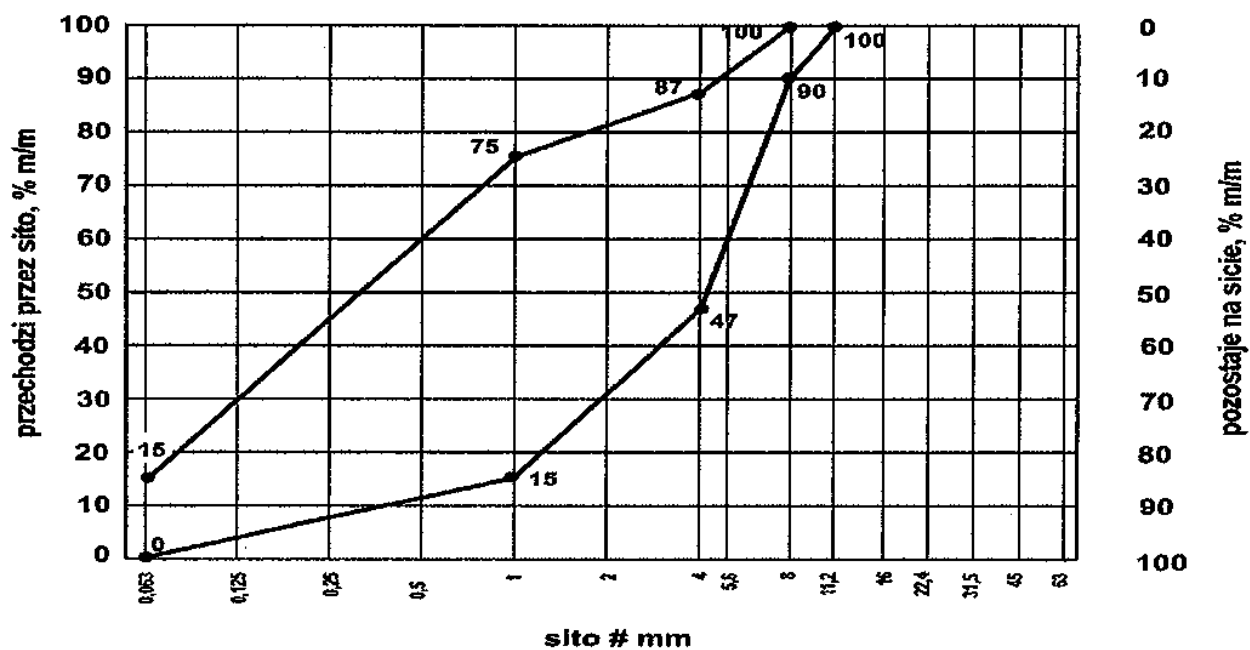
Rys. 6 Mieszanka 0/22,4
