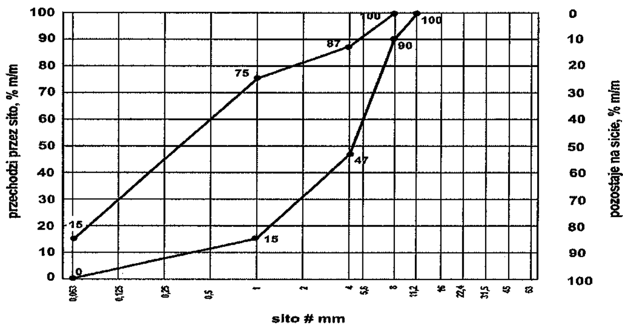
Rys. 8 Mieszanka 0/45
