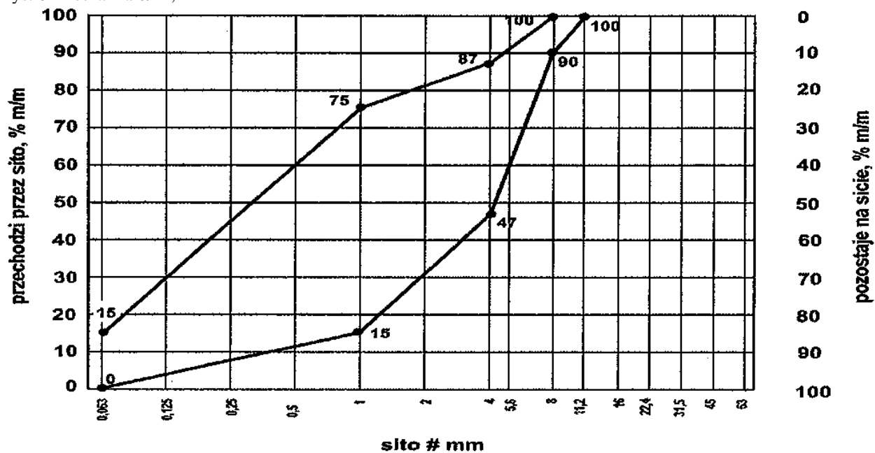
Rys. 7 Mieszanka 0/31,5
