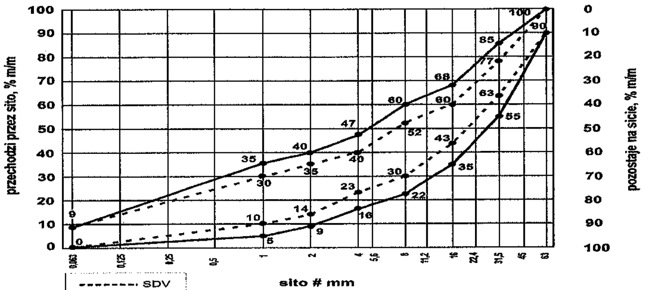
Rys 2 Mieszanka niezwiązana 0/63
