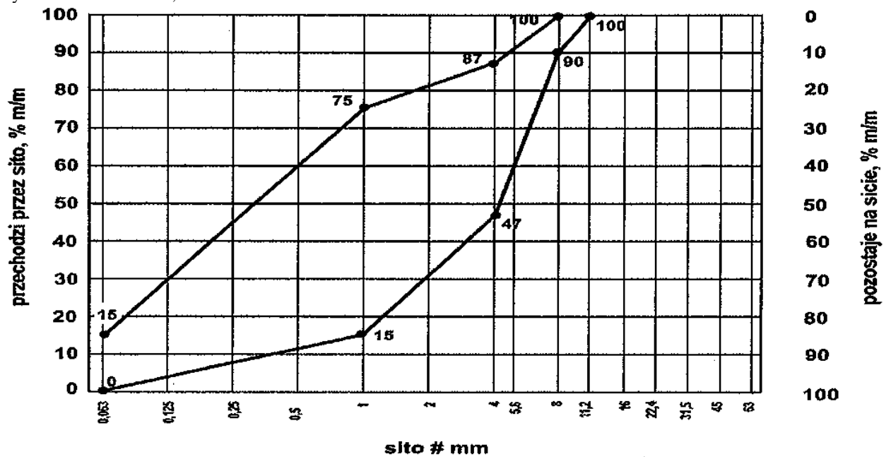
Rys. 5 Mieszanka 0/16
