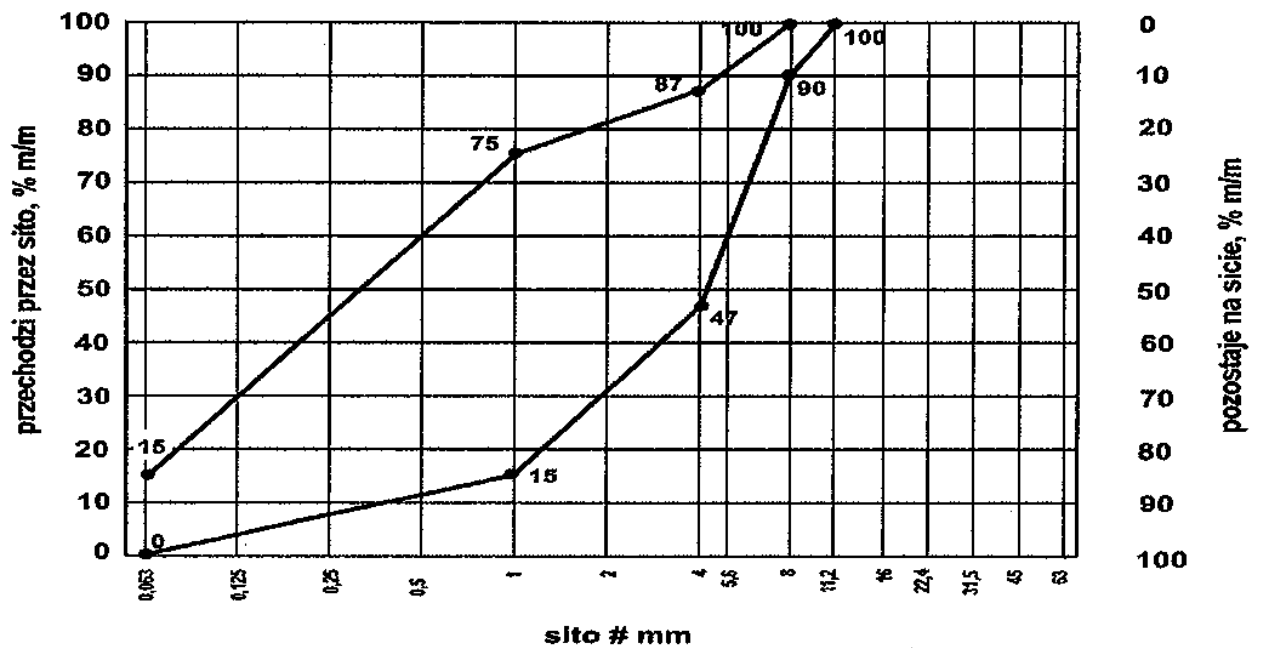
Rys. 4 Mieszanka 0/11,2
