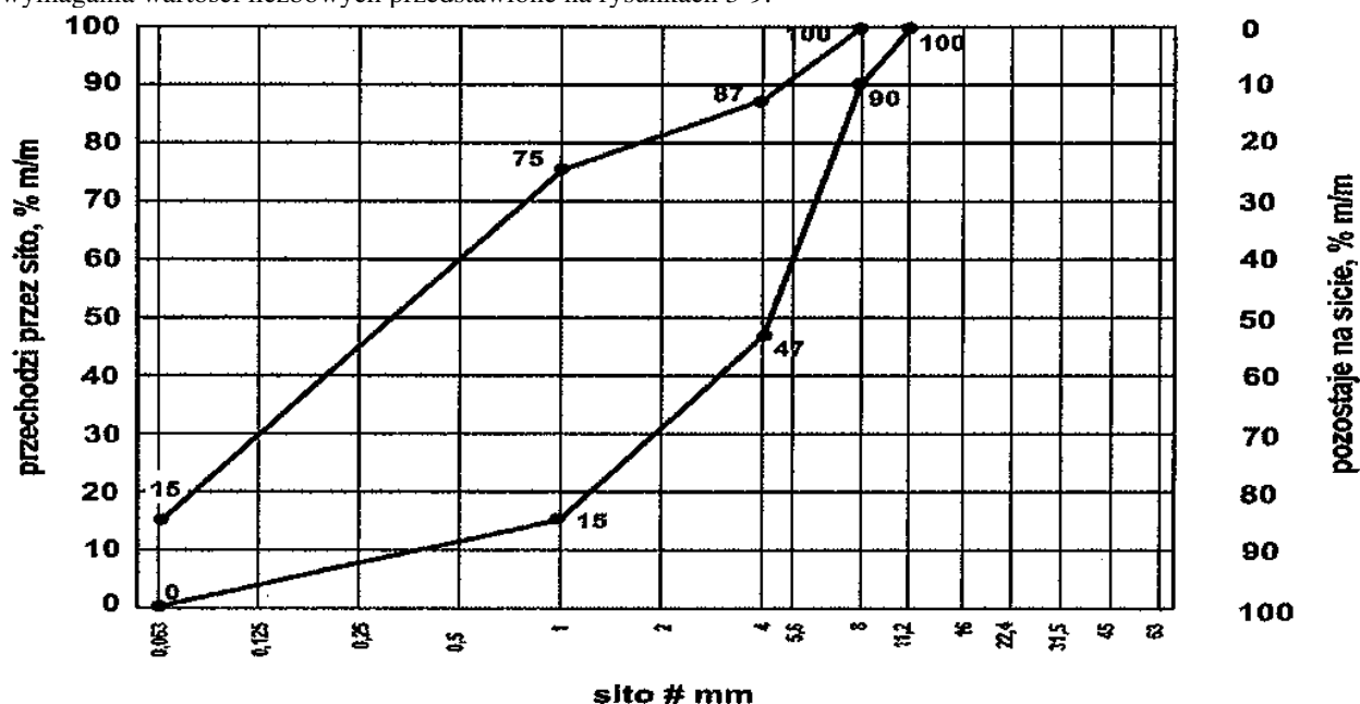
Rys. 3 Mieszanka 0/8
