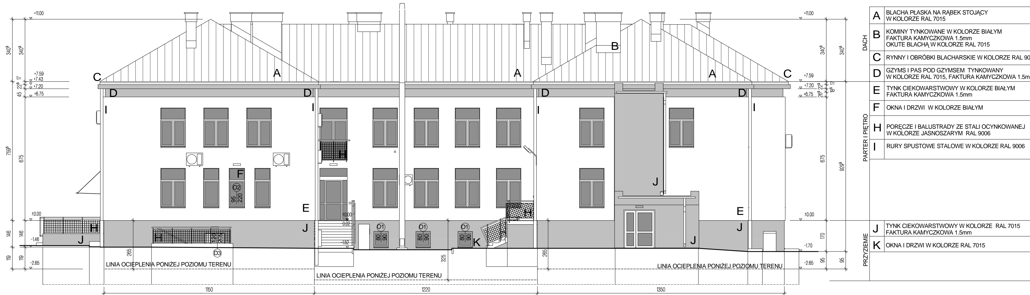
ELEWACJA ZACHODNIA
