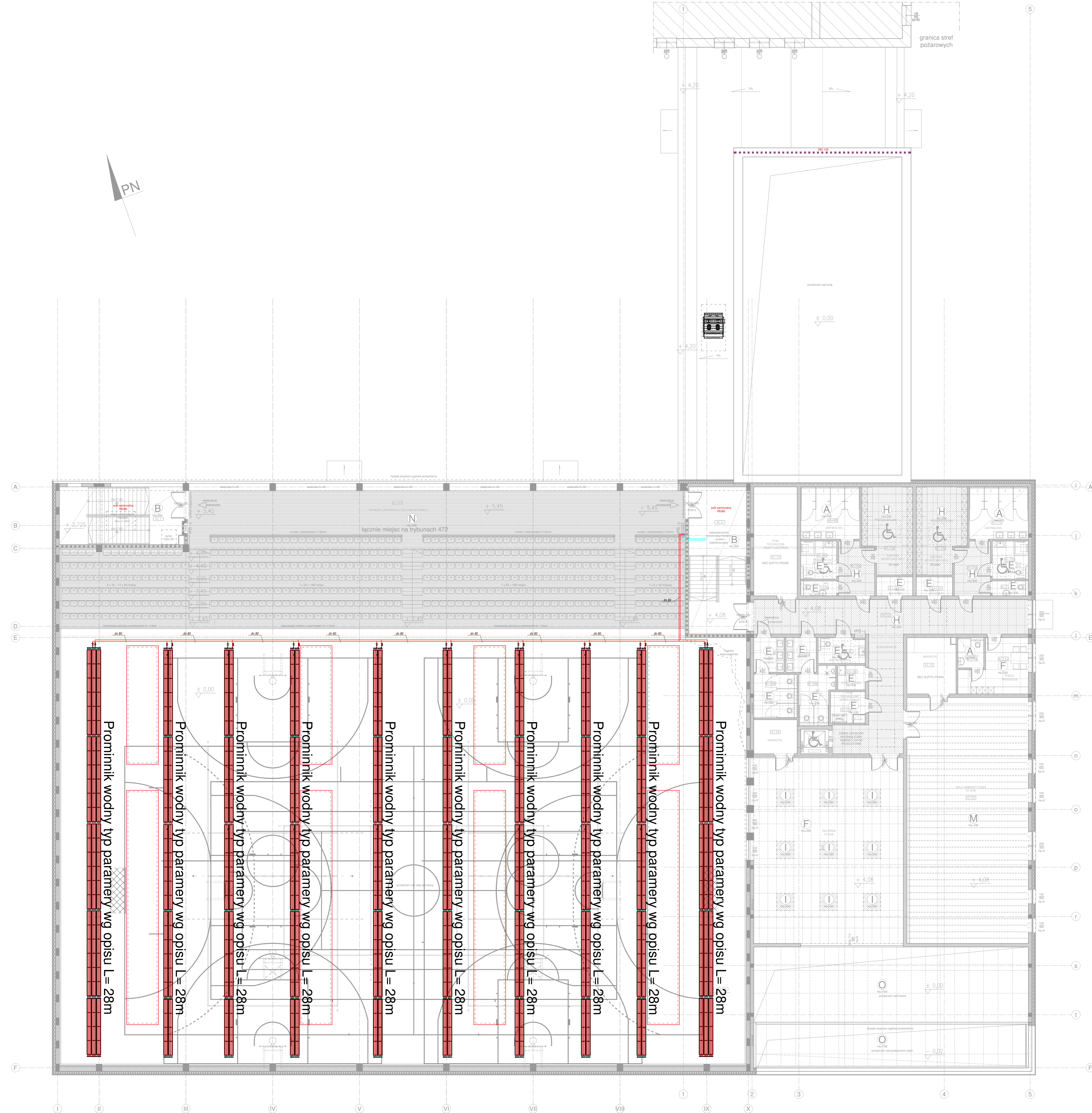
Promiennik Wodne Rzut Skala 1:100
