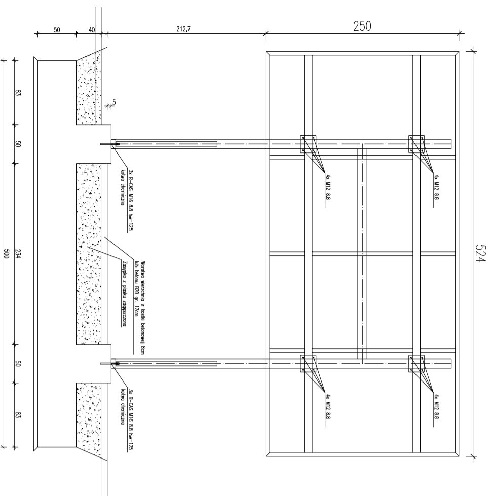
WIDOK OD TABLICZY
