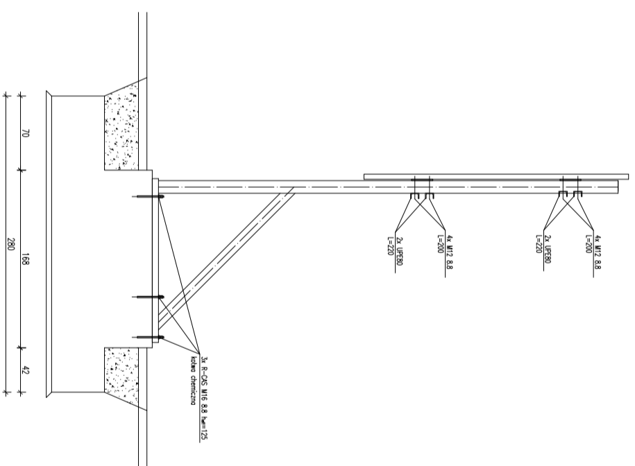
WIDOK Z BOKU MONTAŻ JEDNEJ TABLICZY
