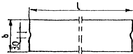
Rys. 1. Wymiarowanie krawężników
