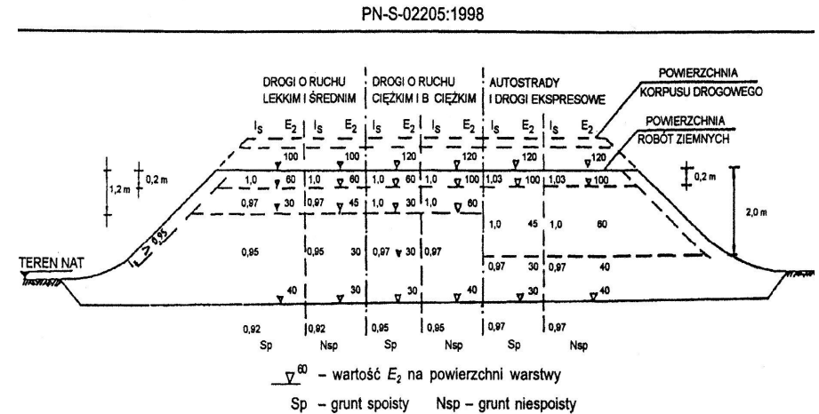
Rysunek 3 - Wartości wymagane w nasypach: wskaźnika zagęszczenia I_s i wtórnego modułu odkształcenia E_2 , megapaskali
