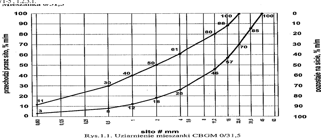
Rys.1.1. Uziarnienie mieszanki CBGM 0/31,5
