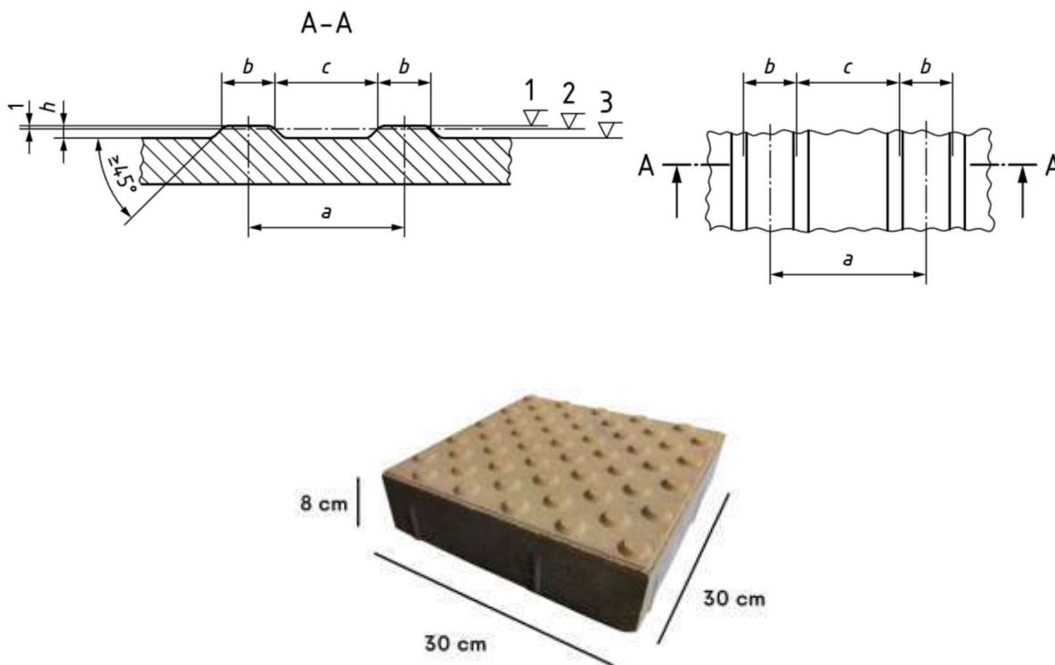
Rys. 2a. Płytki ostrzegawcze (pole decyzji)
