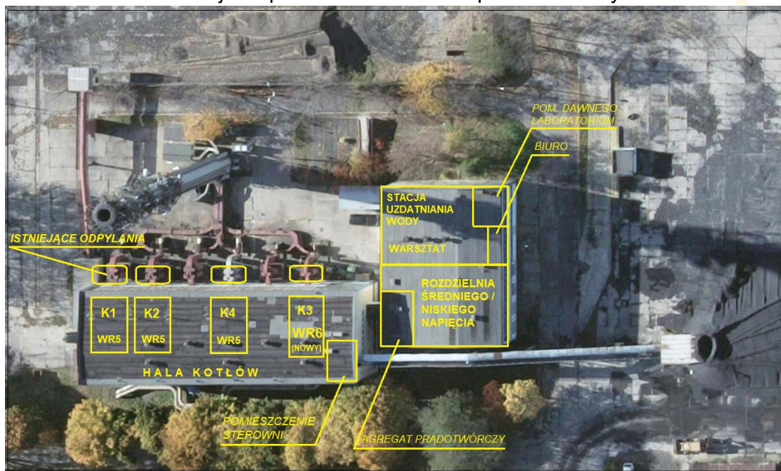
Rysunek 7. Schemat rozmieszczenia urządzeń kotłownia CO 2
