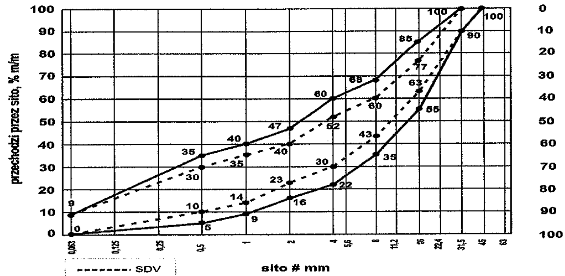
Rysunek 4. Mieszanka kruszyw 0/31,5 do warstw podbudowy zasadniczej
