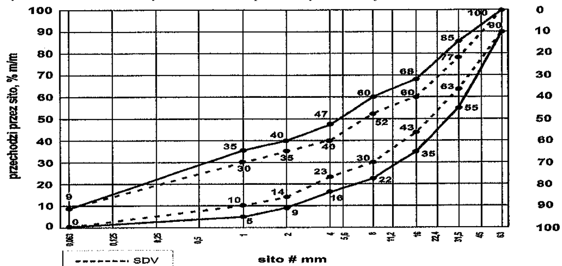
Rysunek 5. Mieszanka kruszyw 0/63 do warstw podbudowy zasadniczej
