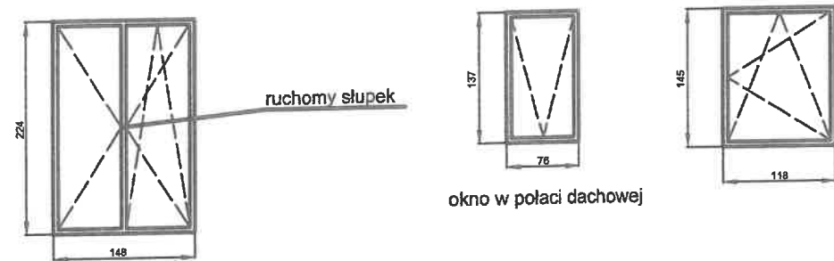
drzwi balkonowe
