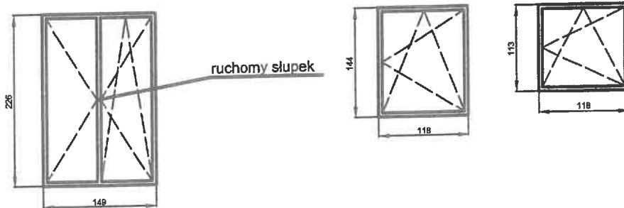
drzwi balkonowe
