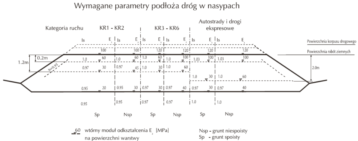
Rys. nr 1 Wymagane parametry podłoża dróg
