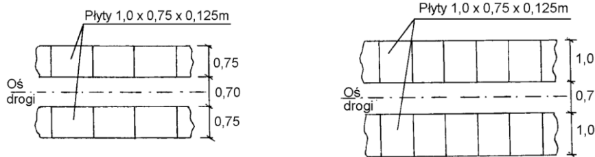
Rys. 2. Przykłady ułożenia płyt na jezdni jednopasowej
