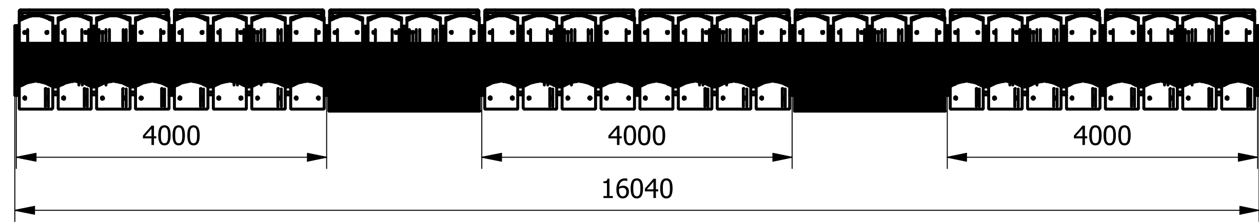
Trybuna rzut 1:50
