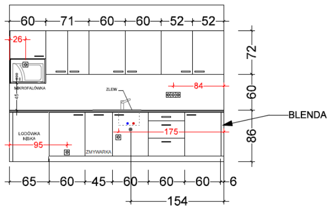
2. WIDOK A-B
