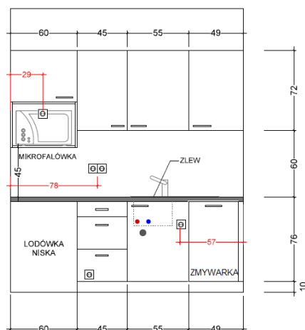
1. WIDOK A-B
