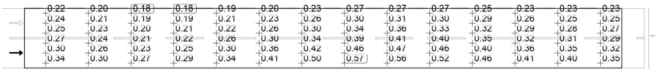
Obserwator 1: Wartości konserwacji, luminacja przy suchej jezdni [cd/m 2 ] (Izoluxy)
