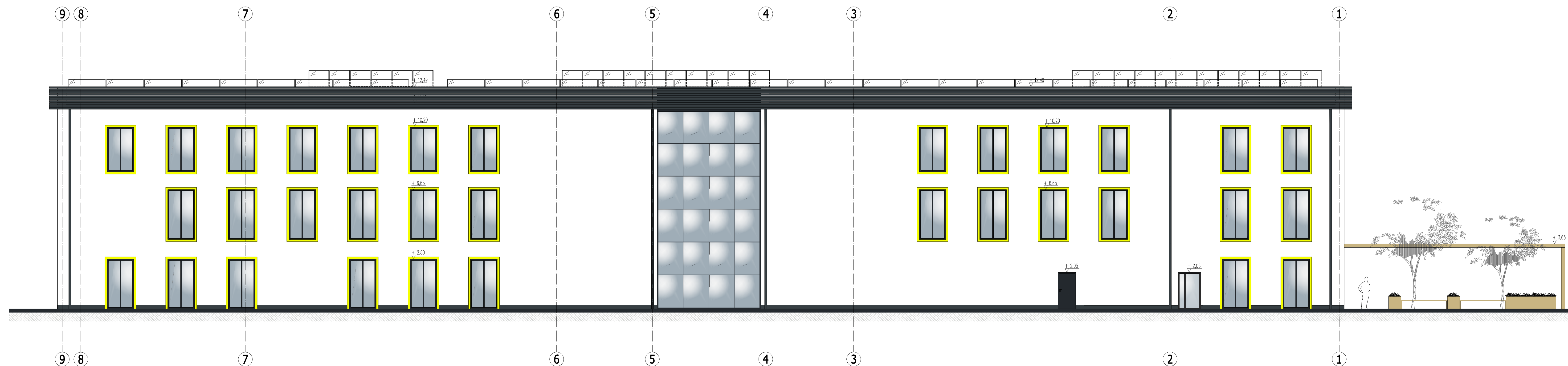
ELEVACJA PÓŁNOCNA
