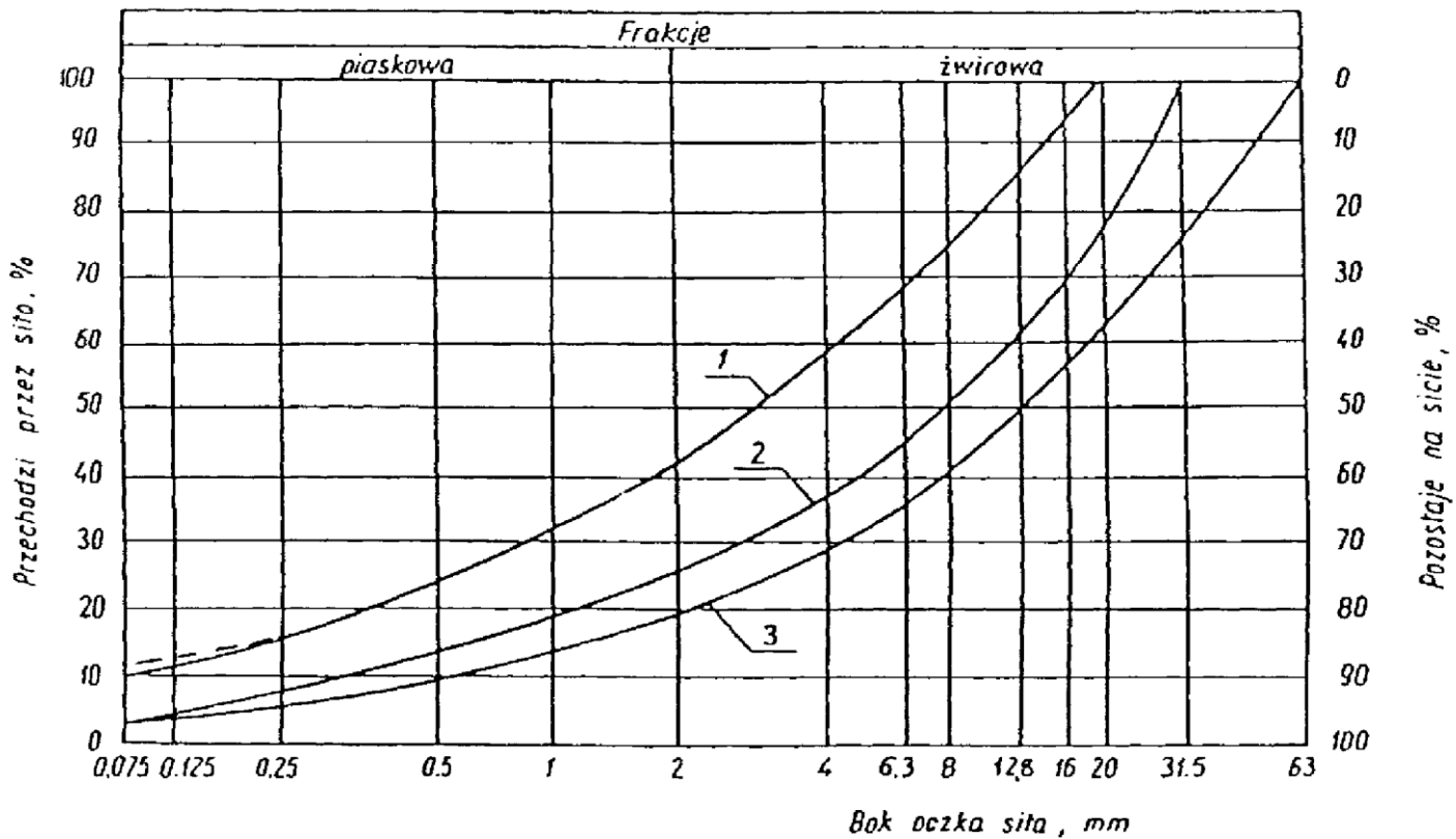
Rysunek 1. Pole dobrego uziarnienia kruszyw przeznaczonych na podbudowy wykonywane metodą stabilizacji mechanicznej 1-3 kruszywo na podbudowę pomocniczą (dolną warstwę) 0-31,5 mm Krzywa uziarnienia kruszywa powinna być ciągła i nie może przebiegać od dolnej krzywej granicznej uziarnienia do górnej krzywej granicznej uziarnienia na sąsiednich sitach. Wymiar największego ziarna kruszywa nie może przekraczać 2/3 grubości warstwy układanej jednorazowo. 2.3.2. Właściwości kruszywa
