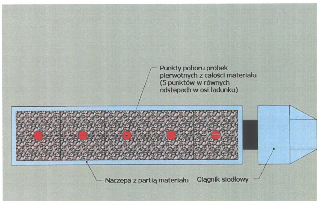
Pobieranie próbek pierwotnych z naczepy pojazdu
