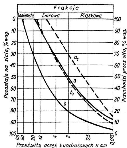
Rysunek 1. Obszar uziarnienia optymalnych mieszanki żwirowych
